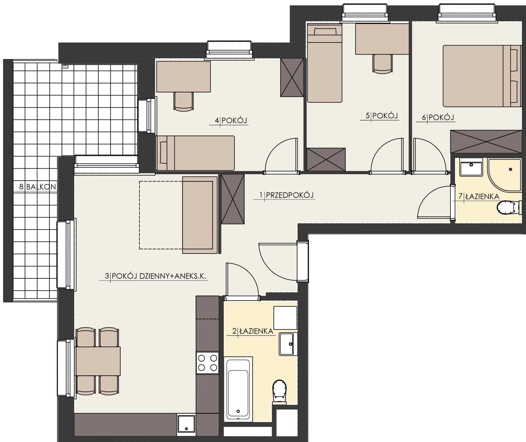
RZUT PIĘTRA 1
