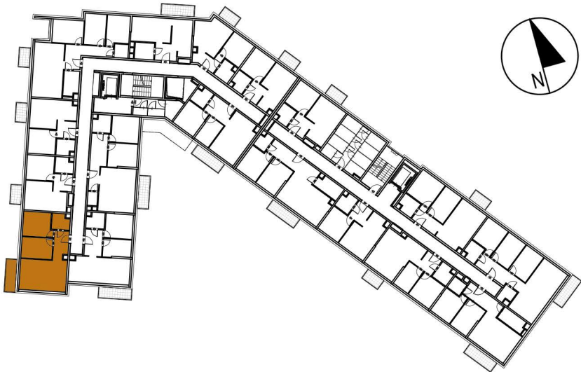
RZUT PIĘTRA 1
